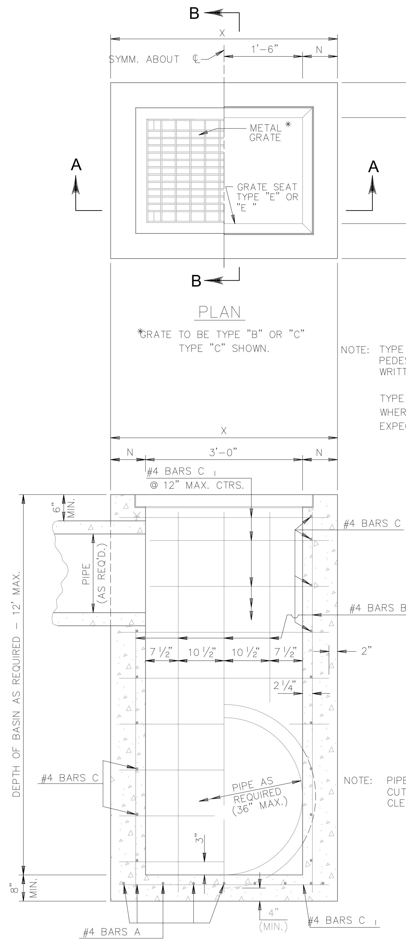
SECTION A-A
